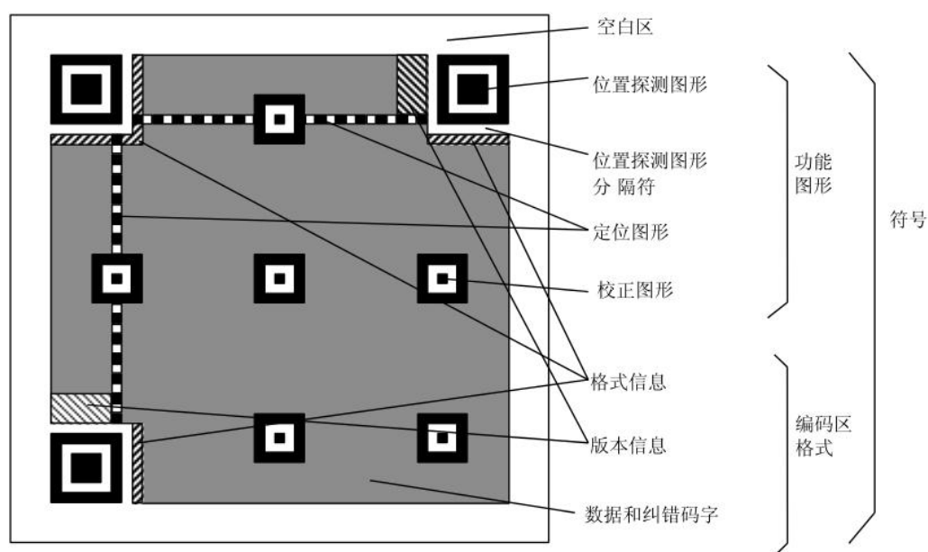
图 1 QR 码的符号结构
