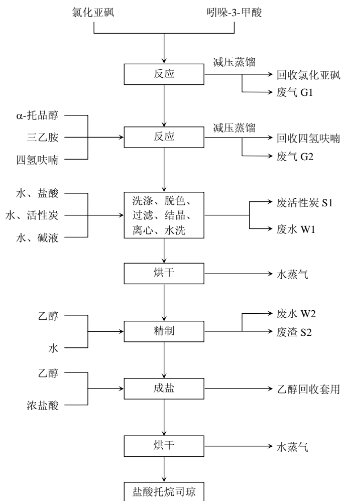
图 B.1 盐酸托烷司琼带产污节点的工艺流程图
